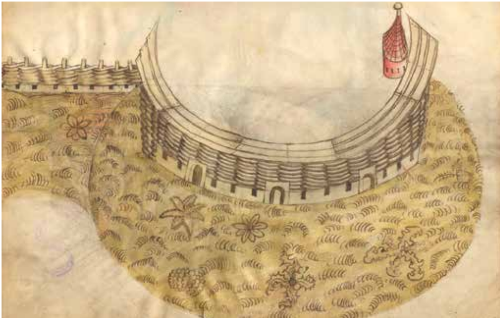
6 Twee tekeningen uit het Kriegsbuch van Ludwig von Eyb uit 1509, blad cr en cv. Het gelegenheidsbolwerk of de schans is zowel vanbuiten als vanbinnen weergegeven. De constructie van houten pijlers en vlechtwerk van takken is goed zichtbaar.
