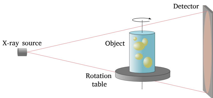
Figuur S2: Een voorbeeld CT opstelling die men in vaak in laboratoria aantreft.
