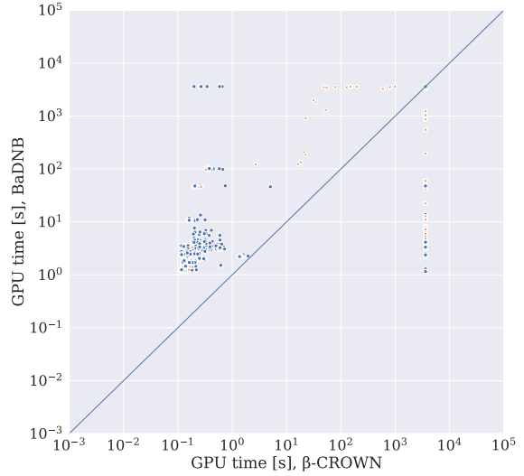
(d) GPU - CIFAR
