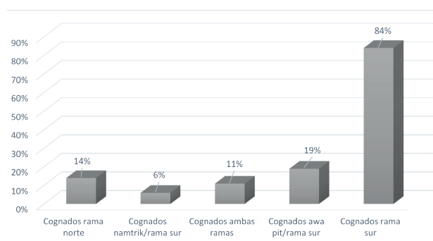
Gráfico 2. Porcentaje de cognados en las ramas de la familia barbacoa.
