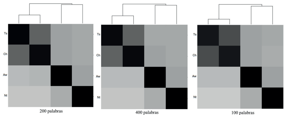
Gráfico 4. Cognados con 100, 200 y 466 palabras.
