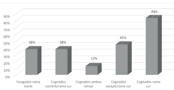
Gráfico 3. Porcentaje de cognados entre ramas de la familia barbacoa en la lista de Swadesh.
