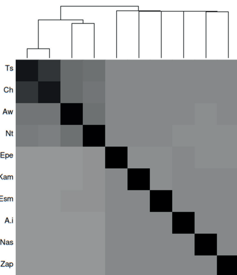
Gráfico 6. Estudio de cognados en lenguas de la región.
