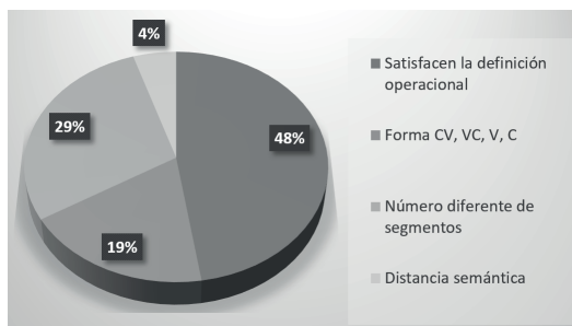
Gráfico 1. Porcentaje cognados según criterios para la definición operacional.
