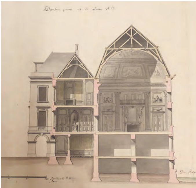
4.11 F.L. Gunckel (1748-1835), 'Doorsnee genome op de Linie AB', 1776. Ontwerp voor de nieuwe vleugel in het Stadhouderskwartier te Den Haag. NA, 4OPG, 1e serie, H299-1. In de kamers links boven (waarschijnlijk een slaapkamer) en de kamer links onder (kabinet?) zijn bespanningen gedacht. Foto: auteur.
