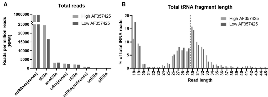
Figure 1. sRNA-seq
