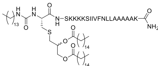
(((2S,5R)-5-amino-6-((2,3-bis(palmitoyloxy)propyl)thio)-1-hydroxy-3,4-dioxohexan-2-yl)amino)-Ser-Lys-Lys-Lys-Lys-Ser-Ile-Ile-Val-Phe-Asn-Leu-Leu-Ala-Ala-Ala-Ala-Ala-Lys-NH 2 (4d)
