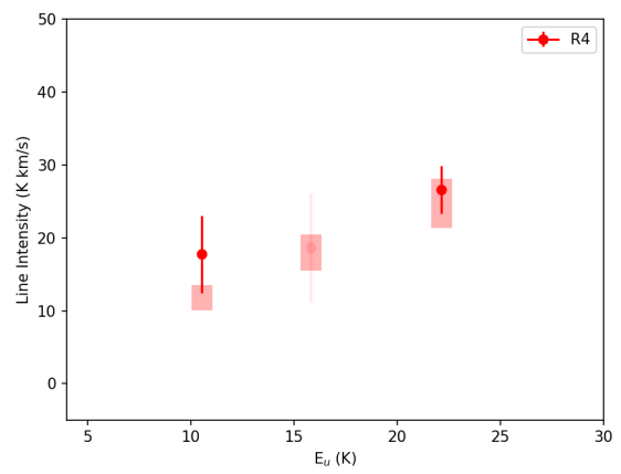
(d) Observed and PPC intensities of HCNCO in CND-R4
