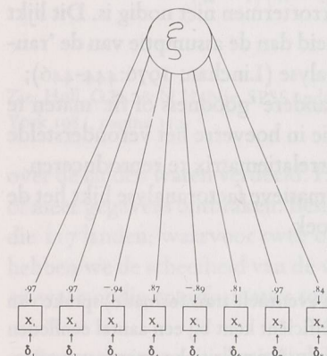
Figuur 1a: Eén-factormodel met ongecorrleerde errortermen
