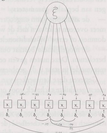
Figuur 1b: Eén-factormodel met gecorrleerde errortermen
