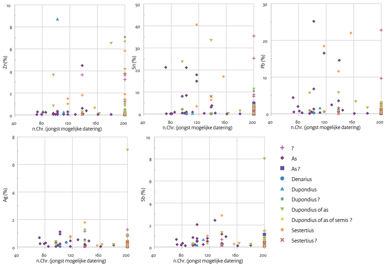
Afb. 6.16 Variatie van legering vormende metalen zink, tin en lood (bovenste rij) en sporenmetalen zilver en antimoon (onderste rij) per munttype (legenda), uitgezet in de tijd van de laatste mogelijke muntslag (x-as). Bij onbekende datum is het jaartal op 200 n.Chr. gezet. De vroegste denarius (consul L. Calpurnius Piso Frugi, muntmagistraat) uit 90 v.Chr. is niet meegenomen.
