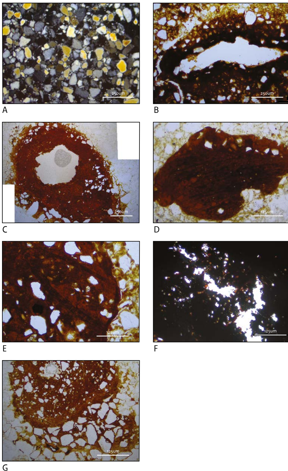
Afbeelding 5.23 Microfoto's uit slijpplaten uit monster 48; zie afb. 5.21 voor de posities in de slijpplaten waar deze foto's vandaan komen. A: Grondmassa van ongesorteerde fijn zand- en siltkorrels (48-2 XPL). B: Donkerrode-zwarte ijzerneerslag in en rondom een porie, lichter gekleurde neerslag in de omringende grondmassa (48-1 PPL). C: IJzerconcretie bestaande uit een holte (waarschijnlijk een oude wortelgang) die deels is ingevuld met ijzeroxides, omringd met door ijzeroxides verkitte grondmassa. De omringende grondmassa vertoont geen ijzerneerslag (48-3 PPL). D: Concretiefragment met restant of afdruk van organisch weefsel ingebed in de ijzeroxide (48-2; PPL). E: Idem. Het organisch weefsel patroon breekt abrupt af op de rand van de concretie, wat een aanwijzing is dat de concretie verplaatst en afgesleten is (48-2; PPL). F: Bewaard gebleven plantaardig weefsel, waarschijnlijk wortelweefsel, in een concretie (48-2; PPL). G: IJzerconcretie waarin meerdere banden herkenbaar zijn met verschillen in ijzermineralogie (verschillende kleuren ijzeroxides) en verschillende groottes in de ingebedde sedimentkorrels (48-3; PPL).
