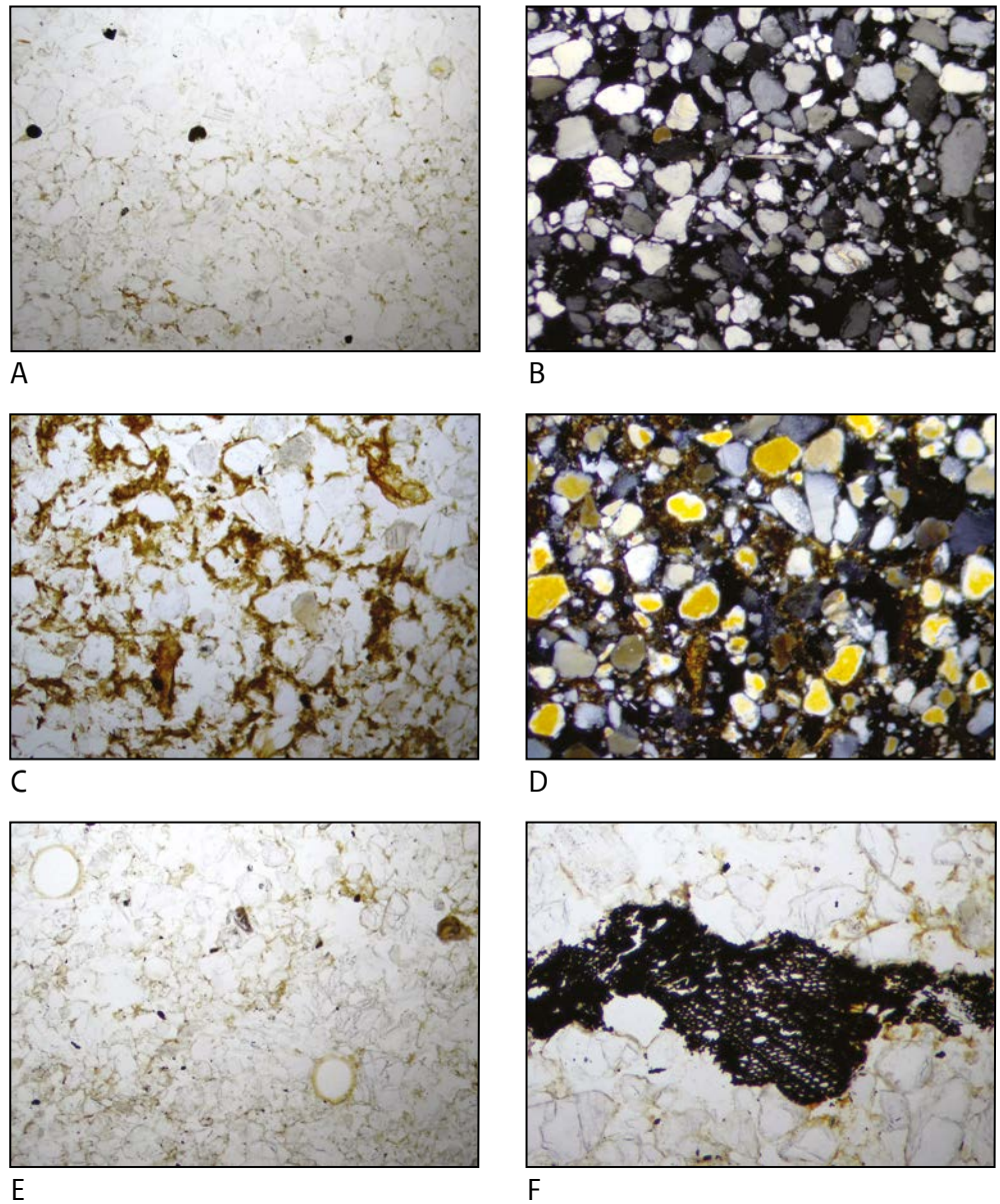
Afbeelding 5.24 Microfoto van fenomenen in de slijpplaten van monster 51. De posities van de foto's in de slijpplaten is weergegeven in afb. 5.22. A, B: Grens tussen fijner (onder) en grover sediment (boven). Binnen het fijnere sediment is geen sortering te herkennen (51-3 PPL, XPL). C, D: Grondmassa met slecht gesorteerde korrels met gelaagdheid die vooral ontstaan door verschillen in organisch stof gehaltes en kleine hoeveelheden klei (51-2 PPL, XPL). E: Fragment verkoold materiaal (51-1, PPL). F: Grondmassa met niet-gelaagde organische resten en twee zaadjes of pollenkorrels (51-1, PPL).
