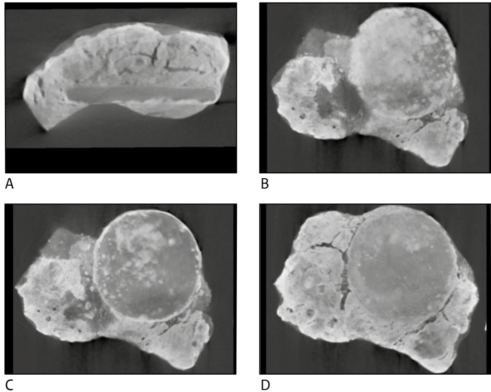
Afb 5.29 Verschillende virtuele doorsnedes door de munt en concretie, en mogelijke interpretatie van de beelden. A: Doorsnede haaks op de munt. De munt is duidelijk zichtbaar als donker deel in de concretie. Met name aan de onderkant is zichtbaar dat delen van de munt zijn omgezet naar een corrosieproduct. B: Doorsnede parallel aan de munt. Onderaan lijken enkele letters zichtbaar te zijn. C: Idem, de witte vlekken vertegenwoordigen mogelijk een zittend figuur. D: Idem (andere kant van de munt). De iets donkerder vlek in het midden is waarschijnlijk een keizershoofd.
