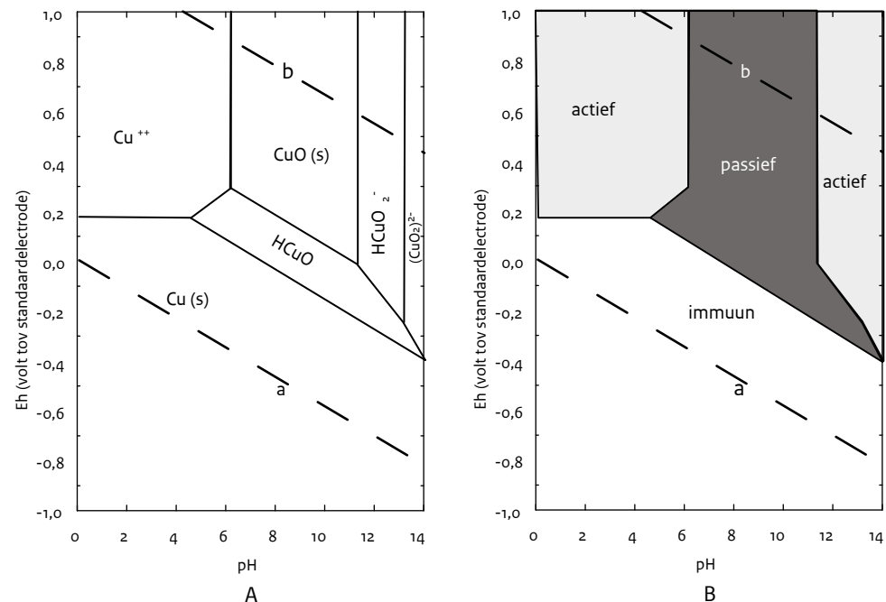
Afb. 7.1 Pourbaix diagram (Eh-pH) van een koper-water-systeem (25 C, 1 atm, \text{Cu}^{2+} = 1 \times 10^{-6} \text{ M} ) naar Selwyn (2004). A: Dit diagram geeft aan onder welke redox- en zuurtegraad condities de verschillende fasen van koper, zuurstof en waterstof stabiel zijn in de bodem. Gebieden zijn gelabeld met de thermodynamisch stabiele species (fase) in dat gebied. Het stabiliteitsgebied van het water is weergegeven door de stippellijn (a en b). Boven lijn b valt water uiteen in zuurstofgas, onder stippellijn a ontstaat waterstofgas. B: Zelfde Eh-pH-diagram, maar nu aangegeven of de species actief (oplosbaar), passief (vaste stof) of immuun (inert; reageert niet) zijn. De stabiliteitsvelden van malachiet en azuriet ( \text{Cu}_2(\text{CO}_3)(\text{OH})_2 en \text{Cu}_3(\text{CO}_3)_2(\text{OH})_2 ) liggen in geval \text{CO}_2 aanwezig is (zoals in de bodem) in het veld \text{CuO} (passief). Goed te zien is dat bij een pH lager dan 6 de stabiele koperoxide fase in een geoxideerde bodem ( \text{Eh} > 0,2 \text{ V} ) overgaat naar een instabiele, actieve opgelost koperfase ( \text{Cu}^{++} ).
