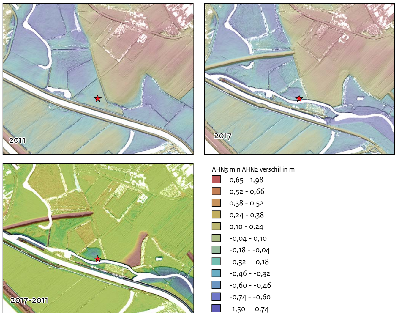
Afb. 2.2 Het Actueel Hoogtebestand Nederland (AHN) versie 2011 (AHN2) en 2017 (AHN3) en een vergelijking tussen de twee versies waarop duidelijk wordt waar afgegraven en opgehoogd is.
