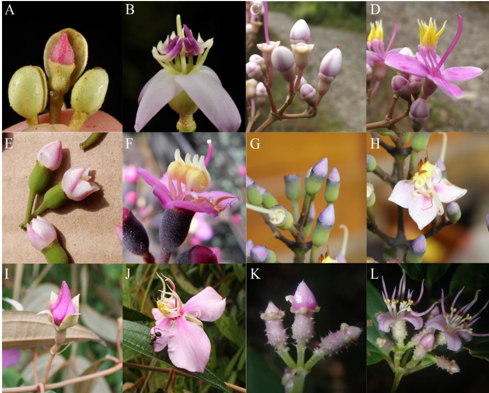
Gbr. 8-4. Kuncup bunga dan bunga masak dari kerabat Dissochaeta . A&B. Creochiton roseus ; C&D. Dissochaeta bakhuiizenii ; E&F. Dalenia glabra ; G&H. Diplectria conica ; I&J. Macrolenes nemorosa ; K&L. Pseudodissochaeta sp. Foto oleh P. Pielser (A&B), A. Kartonegoro (C, D, G, H, I, J), D. Penneys (E&F), M. Nuraliev (K&L).
