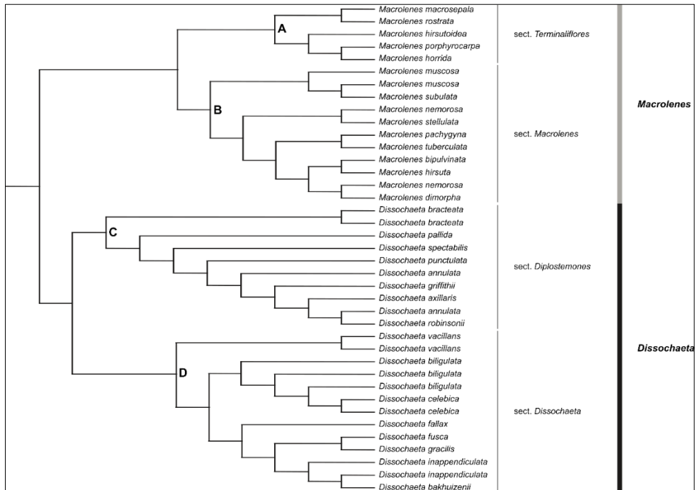
Gbr. 8-6. Pohon filogenetik dari kelompok Macrolenes dan Dissochaeta menunjukkan klasifikasi anak marga baru dalam beberapa seksi.
