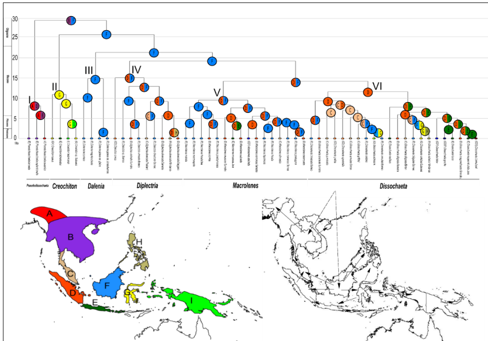
Gbr. 8-7. Kemungkinan area leluhur dan rute penyebaran kerabat Dissochaeta . Warna pada diagram lingkaran dan peta sesuai dengan wilayah geografis; Ma = jutaan tahun yang lalu. A: Bhutan timur, India Timur Laut dan Myanmar Barat Laut; B: Indochina, termasuk Myanmar Tengah dan Timur, Tiongkok bagian Selatan, Hainan dan Thailand; C: Thailand bagian selatan, Semenanjung Malaya dan Kepulauan Riau; D: Sumatera dan pulau-pulau sekitarnya; E: Jawa dan Kepulauan Sunda Kecil kecuali Sumba, Flores dan Timor; F: Borneo; G: Sulawesi; H: Filipina termasuk Palawan; dan I: Maluku dan New Guinea. Kelompok: I. Pseudodissochaeta ; II. Creochiton ; III. Dalenia ; IV. Diplectria ; V. Macrolenes ; VI. Dissochaeta .
