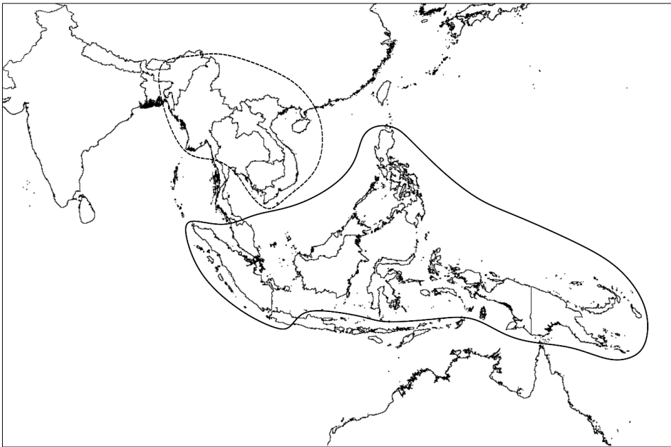
Gbr. 8-2. Peta Distribusi Creochiton (garis bersambung) & Pseudodissochaeta (garis putus-putus).
