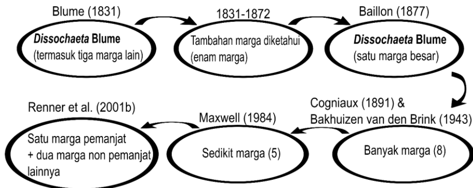
Gbr. 8-1. Ringkasan dan garis waktu dari berbagai batasan marga (= batasan di mana taksa bawahan merupakan bagian dari marga yang dipelajari) dalam kerabat Dissochaeta
