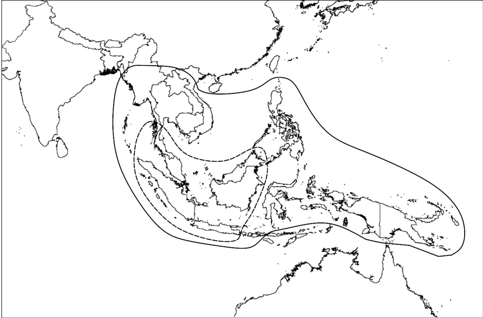
Gbr. 8-3. Peta distribusi Dissochaeta (garis bersambung) & Macrolenes (garis putus-putus).
