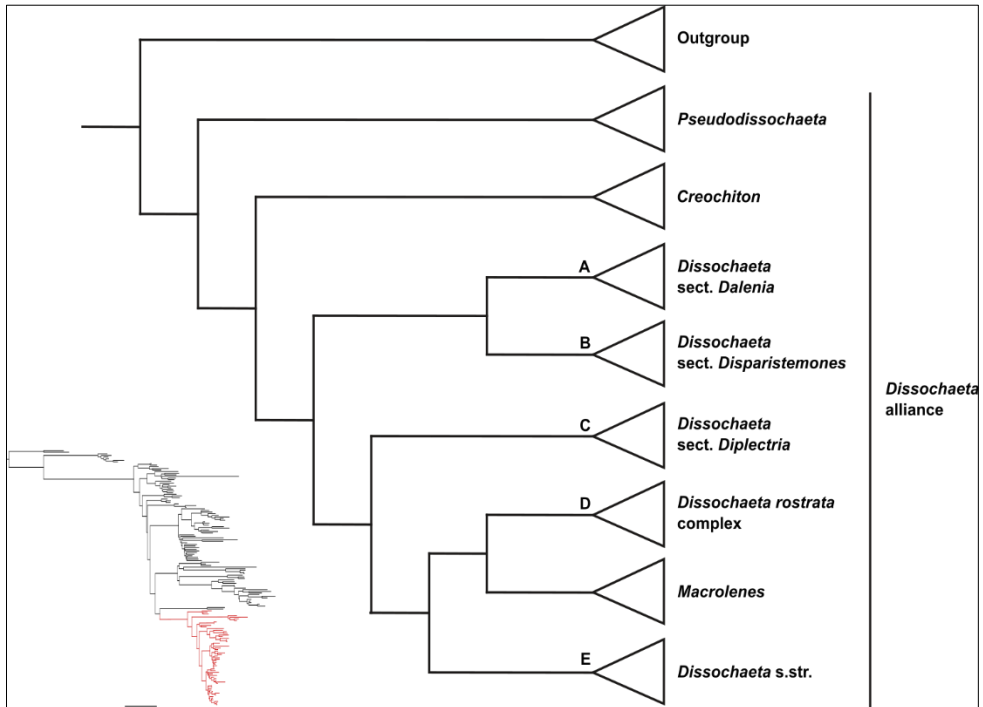
Gbr. 8-5. Pohon filogenetik yang disederhanakan dari kerabat Dissochaeta , di mana segitiga mewakili jenis-jenis. A. Dissochaeta seksi Dalenia (sekarang Dalenia ); B. Dissochaeta seksi Disparistemones (sekarang Dalenia ); C. Dissochaeta seksi Diplectria (sekarang Diplectria ); D. Kompleks Dissochaeta rostrata (sekarang Macrolenes ); E. Dissochaeta s.str. (sekarang Dissochaeta ). Kiri bawah: kladogram dari sampel Melastomataceae lengkap dimana kelompok merah membentuk kerabat Dissochaeta .
