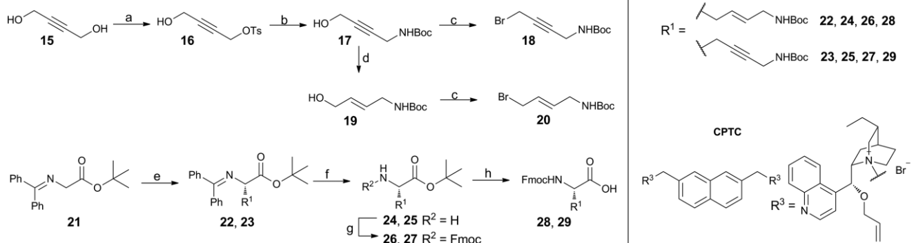
Scheme 1. Synthesis of Lys(4-ene) and Lys(4-yne) building blocks. Reagents and conditions: a) TsCl, pyridine, CH 2 Cl 2 , 63 %; b) 1) NH 3 (25 % aq.); 2) Boc 2 O, Et 3 N, THF, CH 2 Cl 2 , 42 %; c) PPh 3 , CBr 4 , CH 2 Cl 2 , 0 °C; 18 : 68 %, 20 : 58 %; d) LiAlH 4 , THF, Δ, 38 %; e) 18 or 20 , CPTC, toluene/CHCl 3 , KOH (50 % aq.); 22 : 84 %, 79 % ee; 23 : 84 %, 80 % ee; f) citric acid (15 % aq.), THF, 0 °C–r.t.; g) FmocOSu (Fmoc N -hydroxysuccinimide ester), DiPEA (diisopropylethylamine), CH 2 Cl 2 ; 26 : 83 %, 27 : 89 % (over steps f and g); h) 1) TFA; 2) Boc 2 O, DiPEA, MeCN; 28 : 82 %, 29 : 63 %.
