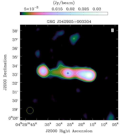
(d) GRG4 (Linear size = 2.40 Mpc)
