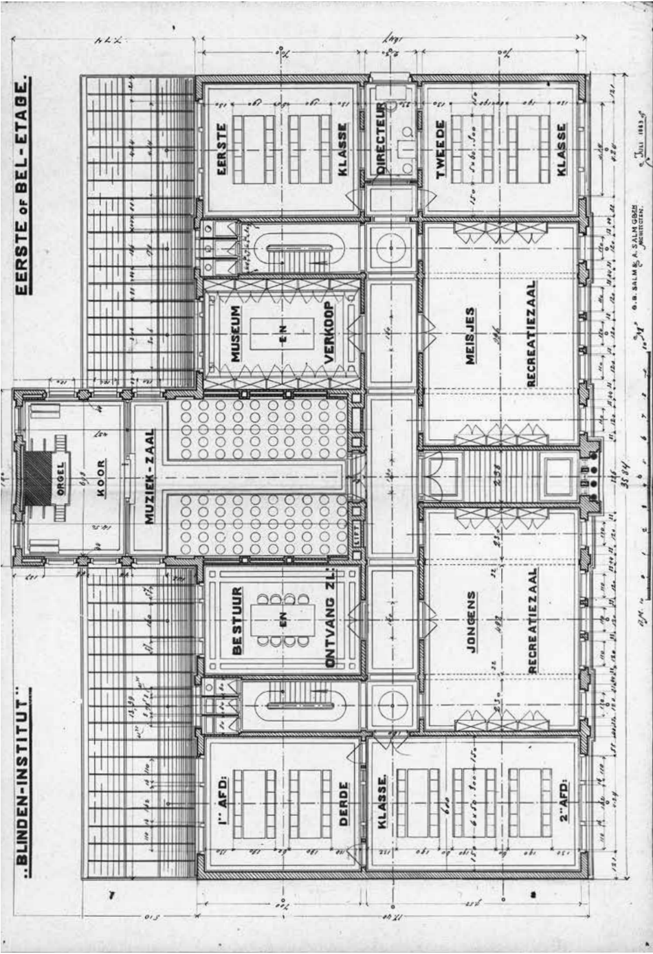
11 B. G.B. Salm en A. Salm, Blindeninstituut (Het instituut tot Onderwijs van Blinden), Vossiusstraat 56, Amsterdam, 1884/1885, bouwtekening eerste verdieping.
