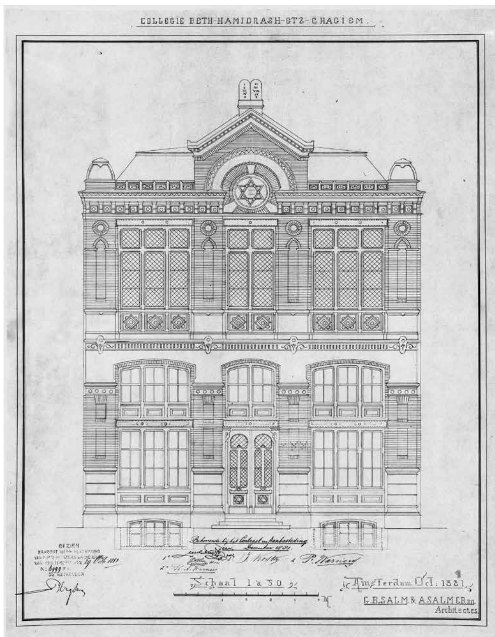
7. G.B. Salm en A. Salm, Synagoge voor het college Beth Hamidrasi Ets Chaïm , ontwerptekening met opstand van de voorgevel, Rapenburgerstraat 109, Amsterdam, 1883.
