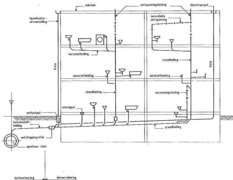
Figuur 1: Benamingen van leidingen
