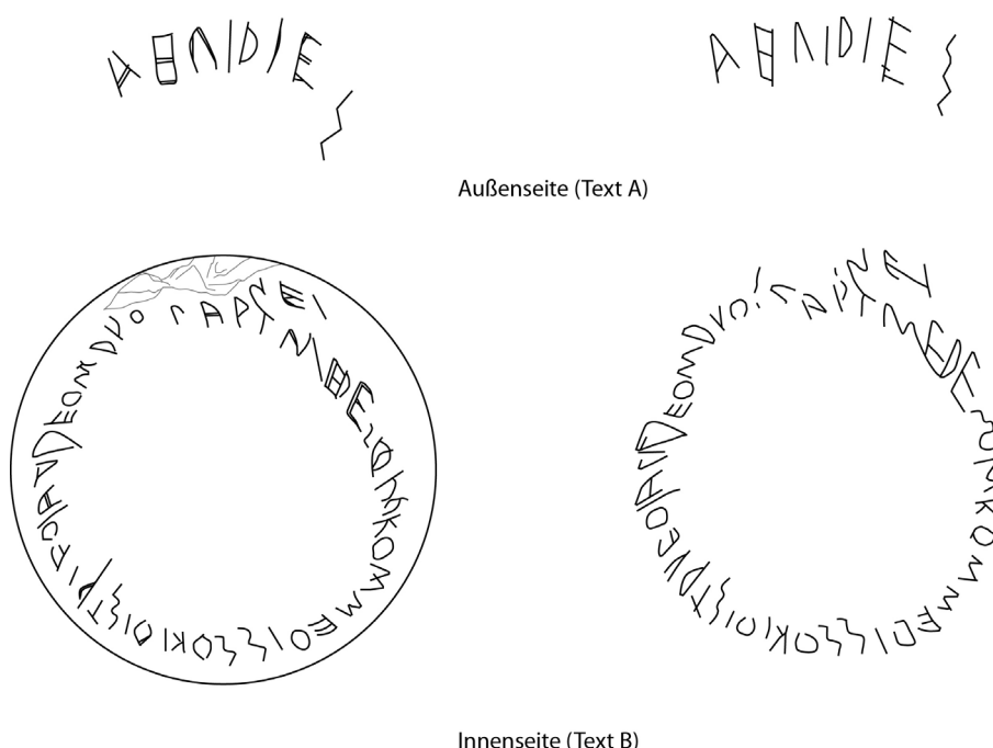
Abb. 5.2: „Garigliano-bowl“ (INS-1), schematische Umzeichnung der Graffiti (links: nach Cristofani 1996, 16 Abb. 9-10; rechts: nach Maras 2005, 35 Abb. 1).
