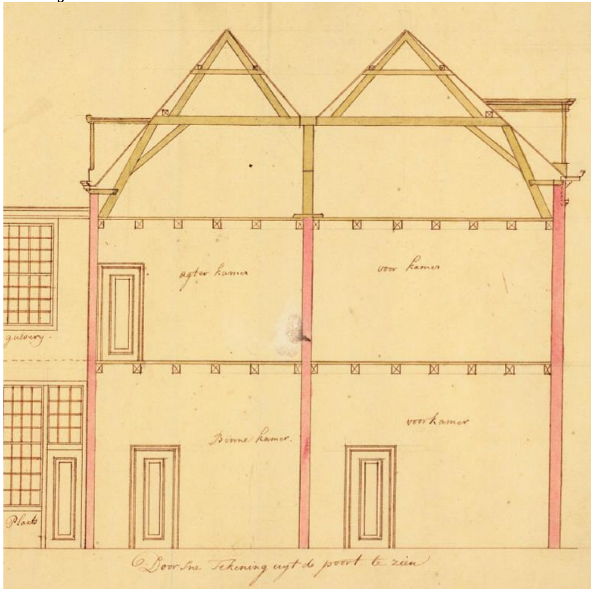
Bouwtekening 1738
