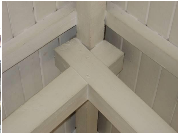
Nokconstructie
