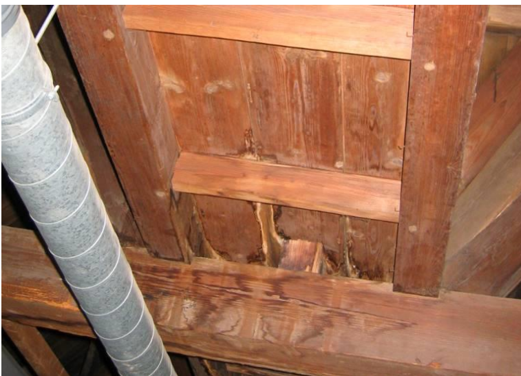
Overzicht gootbodem
