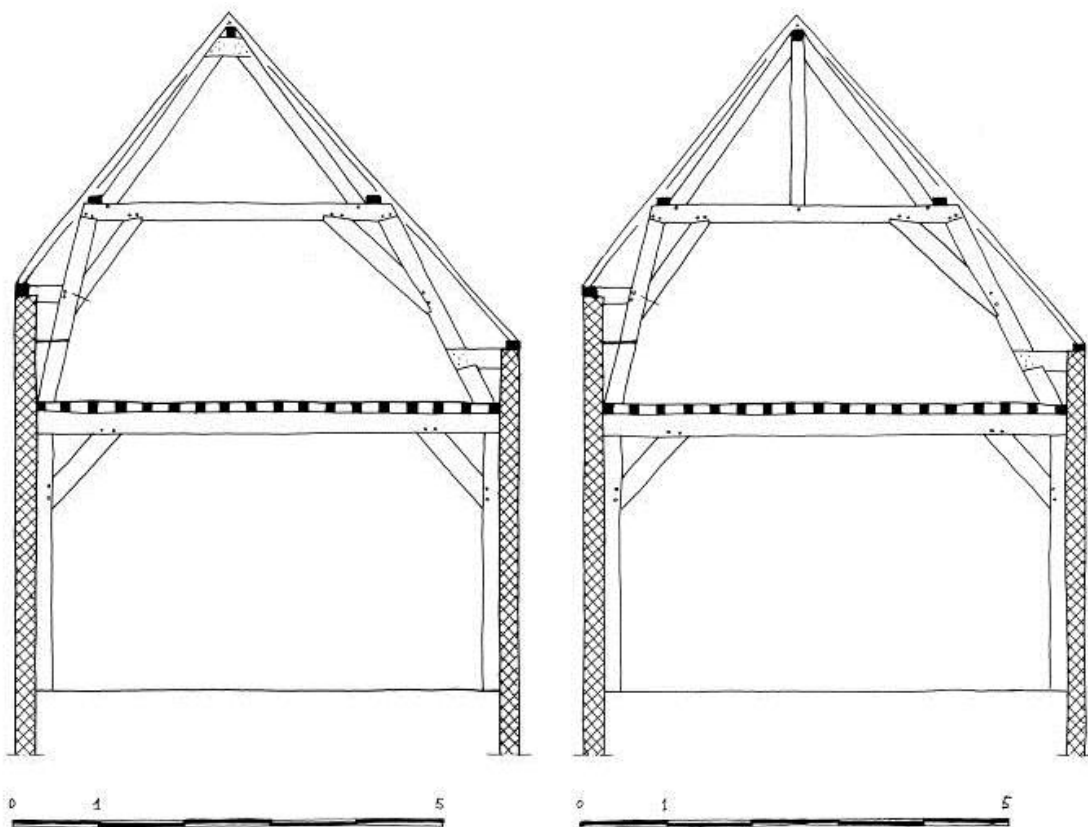
349 en 350 Rapenburg 65, 1749, het ‘normale’ spant (links) en het uiterste spant met makelaar (rechts)
