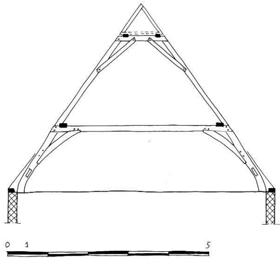
317 Nieuwe Rijn 60, 1404-1416, gelipte korbels
