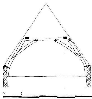
315 Pieterskerkhof 40, 1384, gesmeed blokkeel
