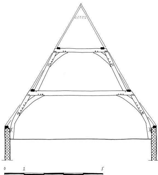
314 Steenschuur 14, 1460-1466, gepend blokkeel
