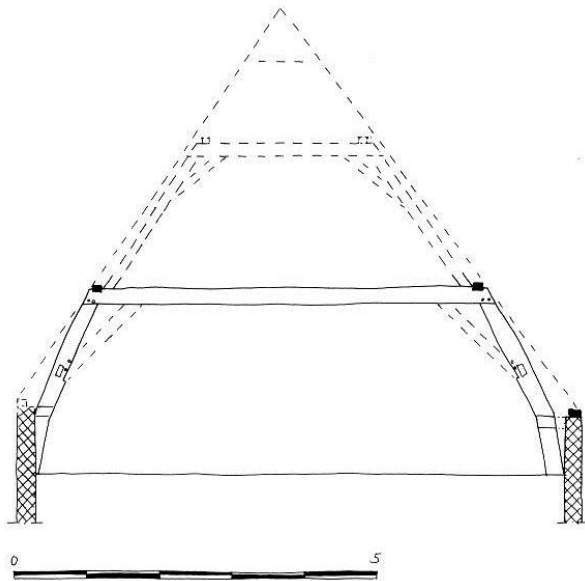
316 Hooigracht 67, 1450, gelipt blokkeel
