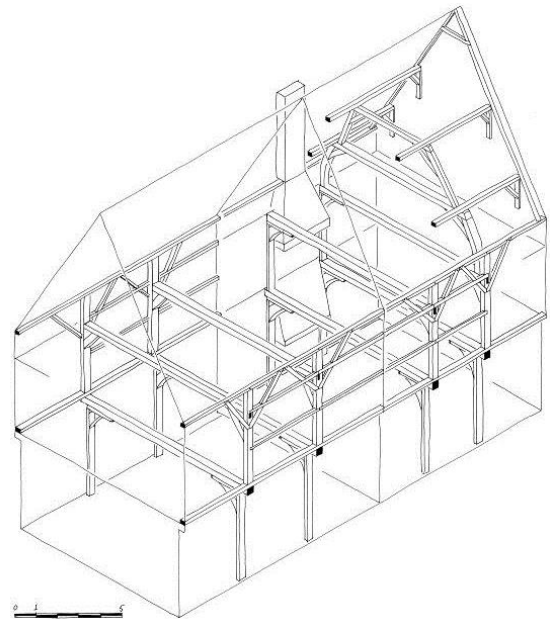
281 Breedstraet 135, 1365, constructieve opbouw
