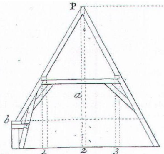
370 Spant met kreupele stijlen (Erzey 1777)
