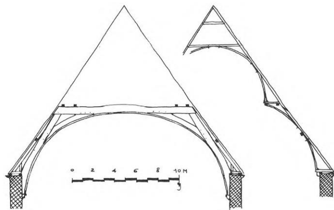
411 Gent, Bijloke, voormalige ziekenzaal, 1251-1255 (d) (Janse 1989)
