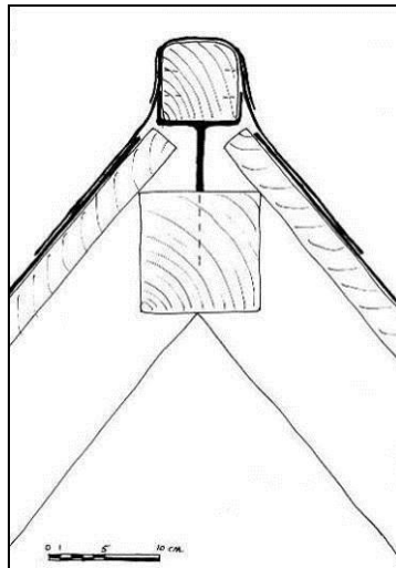
244-245 Nokruiterbokje Rapenburg 67, 1656-1661 (a en d)
