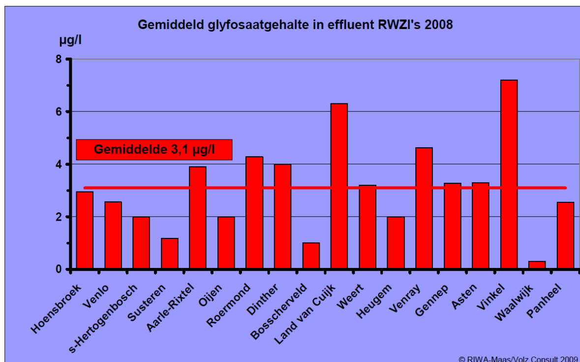
Fig. 4.2.2 Teneur moyenne en glyphosate / Mittlerer Glyphosatgehalt / Average glyphosate concentration 2008
