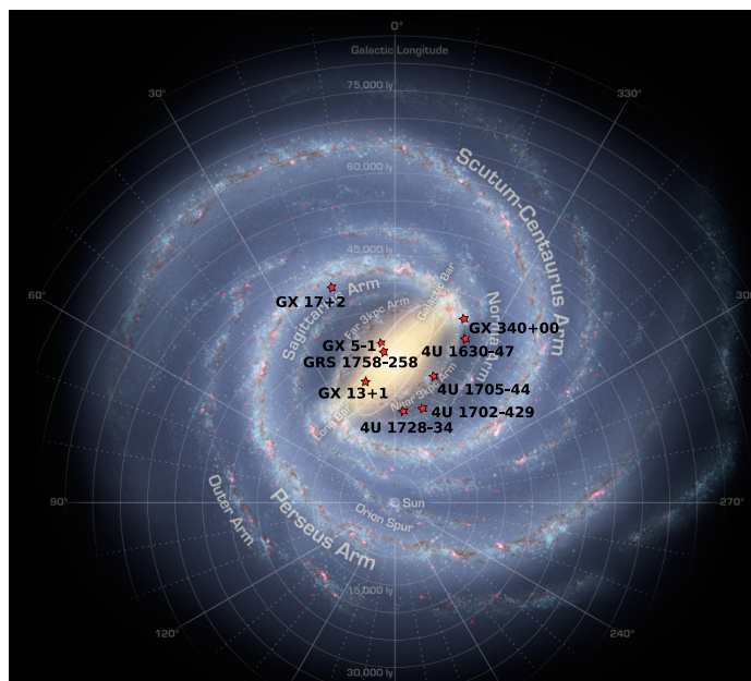
Feguur A.10: Kunstig beêld van een anblik van boven van de Melkweg, maakt nei infraroôdbeêlde van de Spitzer Space Telescope van de NASA. De rooie sterre wiize de plaats an van de LMXB's. © NASA/JPL-Caltech/R. Hurt
