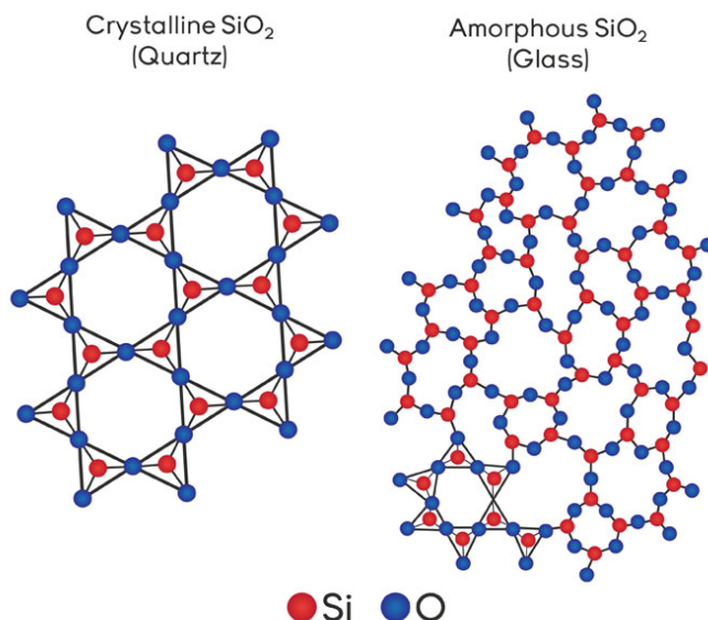
Feguur A.8: Links 't silicaat kwarts, dat een kristallijne structuur heb. Rechts glas met dezelfde atomaire compositie, maar nou zonder de kristalloine geordendhoid van de atome (amorf). In quartz heb elk silicium atoom een band met vier are silicium atome deur "zuurstof bregge". Samen make ze een symmetrische tetraëder. Om niet in de tist te raken, liete we 't vierde silicium atoom en z'n zuurstof breg weg. Bron: NDT Resource Center, Center for NDE, Ioawa State University.
