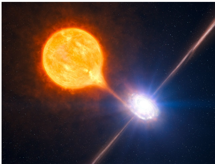
Feguur A.9: Kunstig beeld van een röntgendubbelster, bron: ESO/L. Calçada/M.Kornmesser
