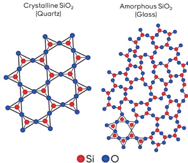
Figuur A.3: Links het silicaat kwarts, dat een kristallijne structuur heeft. Rechts glas met dezelfde atomaire compositie, maar nu zonder de kristallijne geordendheid van de atomen (amorf). In kwarts is ieder silicium atoom verbonden met vier andere silicium atomen via “zuurstof bruggen” en vormt daarmee een symmetrische tetraëder. Voor de duidelijkheid is het vierde silicium atoom en de daarbij behorende zuurstof brug weggelaten. Bron: NDT Resource Center, Center for NDE, Iowa State University.
