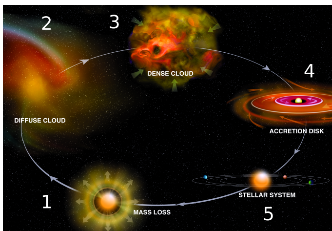
Feguur A.7: De levensloop van sterre en interstellair stof in 5 stadia: 1) geëvolueerde ster, 2) diffuse wolk, 3) dichte wolk, 4) protostellare skoif en 5) stelsel met planete. In alle dêle van stervorming speelt stof een cruciale rol. © Bill Saxton, NRAO/AUI/NSF.
