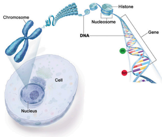
FIGUUR. Structuur van DNA. De chromosomen zijn gelokaliseerd in de celkern en bestaan uit lange DNA-strengen die vele genen bevatten. Chromosomen bevatten eiwitten die histonen worden genoemd, waar het DNA omheen is gebonden. DNA bestaat uit vier componenten die nucleotiden worden genoemd (hier weergegeven in geel, rood, blauw en paars). DNA-methylering (m) en DNA-hydroxymethylering (hm) zijn de weergegeven epigenetische veranderingen [Aangepast overgenomen van TereseWinslow LLC]
