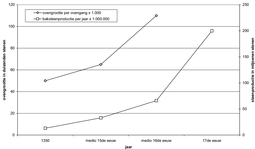
Fig. 10.5 Baksteenindustrie - ovengrootte en steenproductie per jaar
