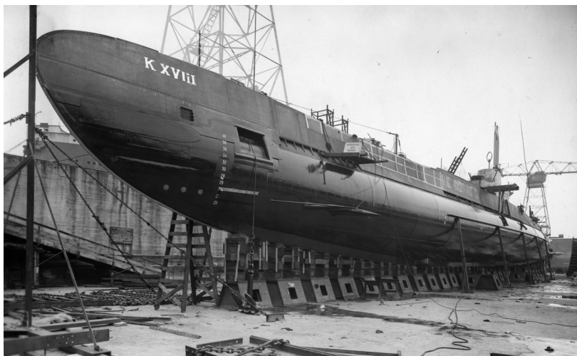
Figuur 6.2 Hr. Ms. onderzeeboot K XVIII in aanbouw bij Feijenoord in Rotterdam. De drie horizontale stippen helemaal onderaan bij de boeg aan bakboord zijn hydrofoons (onderwatermicrofoons). Zij zijn bestemd voor onderwatertelefonie met behulp van geluidssignalen. Hydrofoons, waarvan de boot er aan elke zijde zes bezit, vormen het belangrijkste middel waarmee de onderzeeboot zelfstandig schepen kan opsporen op grotere afstanden. (collectie H.O. Bussemaker)
