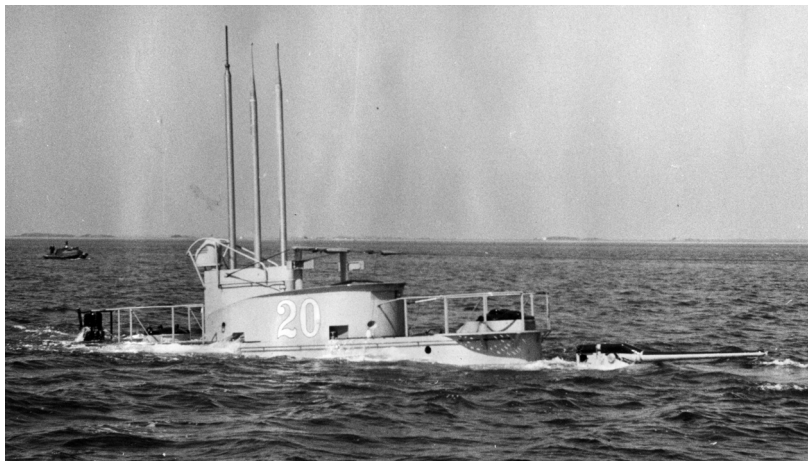
Figuur 7.1 Hr. Ms. onderzeboot O 20 duikt op tijdens proeven in 1939. De hoge 'periscoop' links is de periscoopantenne, eigenlijk een radiomast. De antennestaaf staat er bovenop en is maar een meter hoog. De bolling onder de staaf dient om deze te isoleren. Dankzij de periscoopantenne konden de onderzeeboten onder water verkeningsberichten ontvangen en met elkaar communiceren. Deze Nederlandse uitvinding was veel belangrijker voor hun tactiek dan de snuiver (snorkel), die direct erachter zichtbaar is tussen twee gebogen buizen. Hoewel hier ingetrokken, is de snuiver ook uitgeschoven niet hoog. (Oudere boten voerden op de plaats van de snuiver een in-trekbare mast met radiokabels, die alleen boven water bruikbaar waren.) Rechts van de periscoopantenne staan de twee periscopen, een voor de aanval en een voor de navigatie, welke ook vliegtuigen kan ontdekken. (collectie H.O. Bussemaker)
