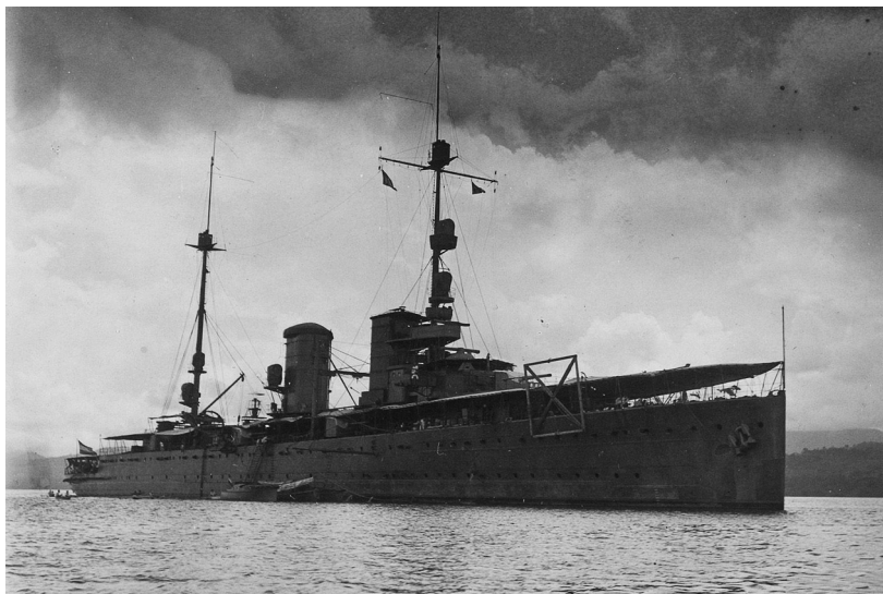
Figuur 6.1 Hr. Ms. Java in april 1926, vermoedelijk voor Ambon. Het voorste kanon staat verscholen onder het tentzeil tegen de tropenzon. Het grote vierkant met een kruis erin naast dit verscholen kanon is het geraamte van een schietschijf. Uiterlijk deed deze door de Duitse Krupp Germaniawerft ontworpen en met hulp van deze werf bij De Schelde in Vlissingen gebouwde lichte kruiser sterk denken aan de (veel sterkere) Duitse slagkruisers. (KITLV signatuur 52642)
