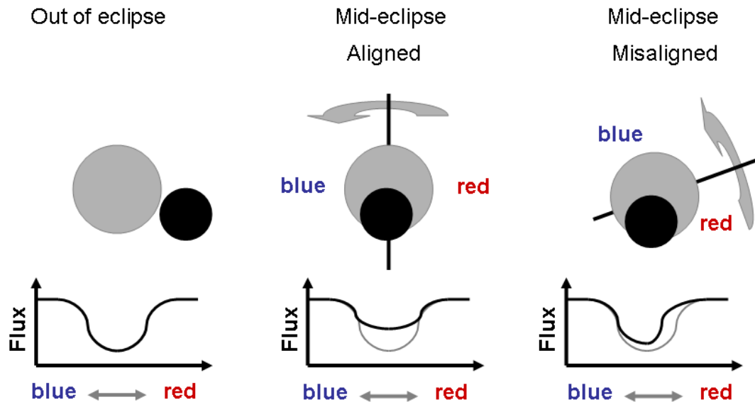
Figuur 7.3 — Schematische voorstelling van het Rossiter-McLaughlin effect. Vanwege het draaien van de ster is een geobserveerde absorptielijn verbreed (links). Een gedeeltelijke verduistering door een object op de voorgrond vervormt de absorptielijn anders als de as een rechte hoek maakt (midden) dan als hij geen rechte hoek maakt (rechts) met het vlak van de baan waarin de sterren zich bewegen.
