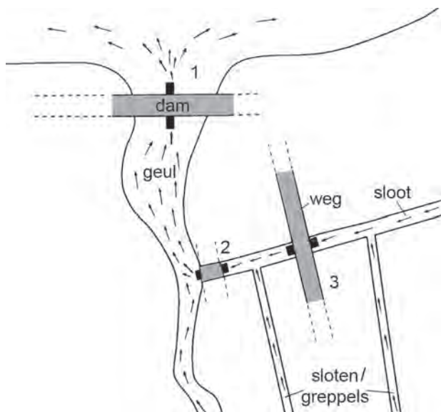
Fig. 5.27. Typen duikers (naar Ter Brugge 2002, 65-66, afb. 3). Het gaat om de uitwateringsduiker met klep, geplaatst in een dam in een geul (1) of sloot (2). Duikers kunnen ook als verbindingsduiker zijn gebruikt (3).
