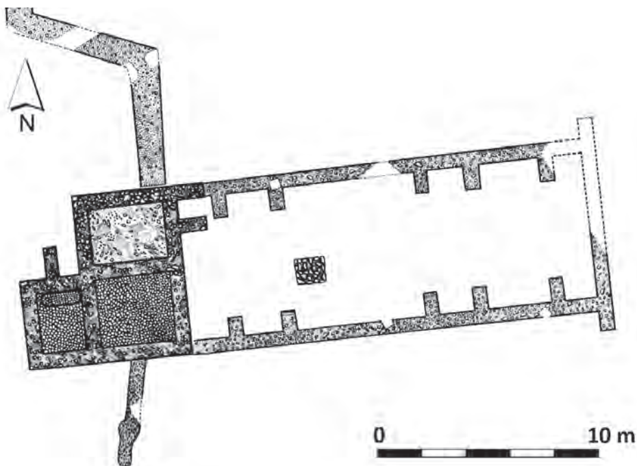
Fig. 5.19. Gebouw met stenen fundering in Rijswijk-De Bult. Naar Bloemers 1978, Beilage 1a.
