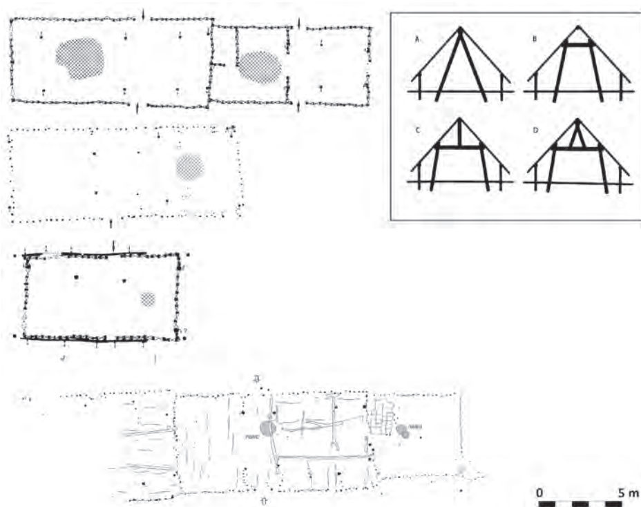
Fig. 5.5. Enkele huisplattegronden uit de microregio Schiedam. Afbeelding naar Hallewas 1986, 49-50, afb. 4, 5 en 6; Meirsman en Moree 2004, 62, afb. 22. Inzet: de A-constructie: A is de traditionele reconstructie en B tot en met D zijn alternatieve constructies (afbeelding en beschrijving naar Kodde 2014, 302, afb. 5).
