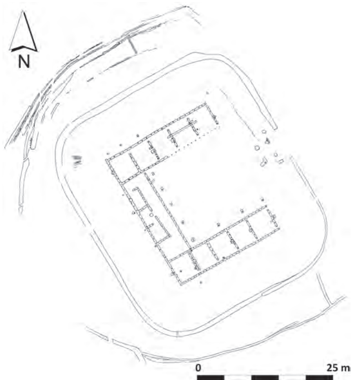
Fig. 3.15. Minicastellum Valkenburg-Marktveld. Het centrale U-vormige gebouw wordt omgeven door een gracht die aan de oostzijde een opening vertoont; hier bevindt zich een poortgebouw. Buiten de gracht bevindt zich een tweede greppel die fragmentarisch bewaard is gebleven. Aan de noordzijde bevinden zich bovendien allerlei stakenrijen. Afbeelding naar tekening G. van Haaff/Rijksdienst voor het Cultureel Erfgoed.
