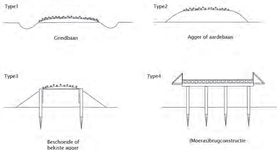
Fig. 3.27. Verschillende typen van de limesweg (naar Luksen-IJtsma 2010, 15, afb. 2.1).
