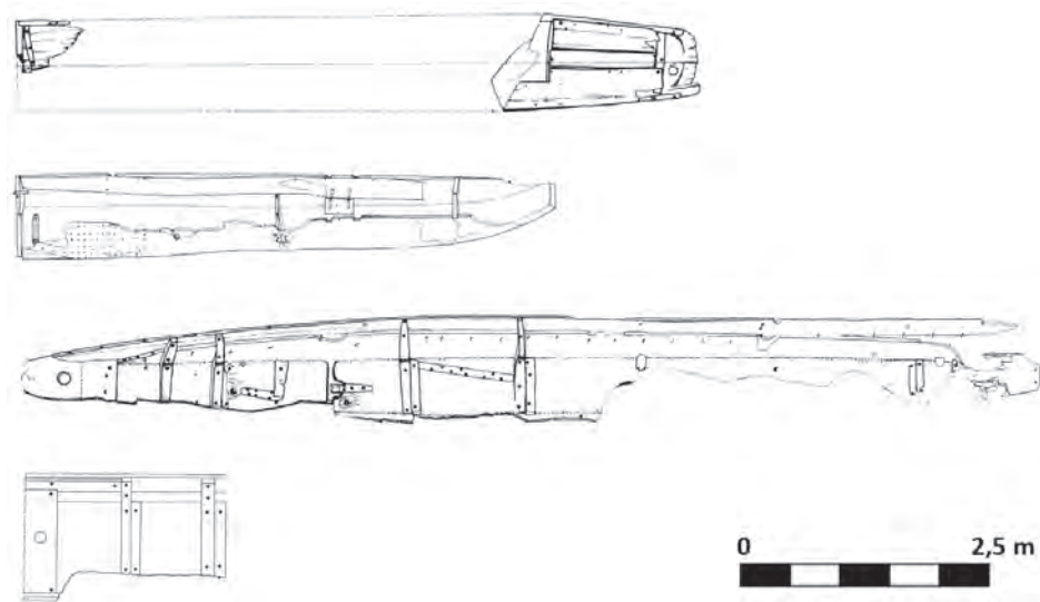
Fig. 3.29. Boomstamboten (bovenste twee, de schepen Zwammerdam 5 en 1) en boomstamplankboten (onderste twee, de schepen Zwammerdam 3 en Woerden 3). Afbeelding naar De Weerd 1988; Hallewas 1989, 338, afb. 16.
