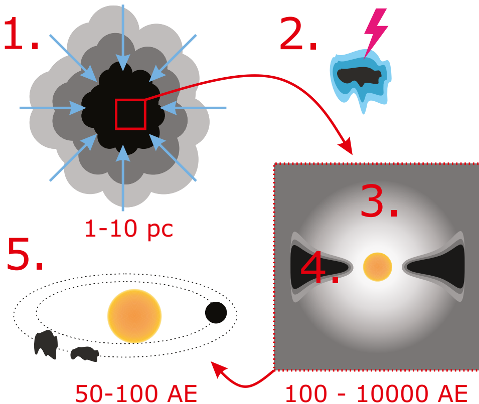
Afbeelding 1. Illustratie van de vorming van een planetenstelsel. Onder invloed van de zwaartekracht stort een interstellaire wolk ineen (1). In de koude regionen vriezen gasmoleculen vast op stofdeeltjes, en in deze ijsmantels kunnen chemische processen plaatsvinden (2). Nadat een protoster gevormd is blijft materie neervallen op de jonge ster. Door de warmte die hierbij vrijkomt verdampen ijsmantels en komen complexe moleculen in de gasfase (3). De invallende materie vormt een protoplanetaire schijf rond de protoster (4), waaruit uiteindelijk kometen en planeten ontstaan (5). 1 AE is de Astronomische Eenheid, de gemiddelde afstand tussen de aarde en de zon, gedefinieerd als 149 597 870,7 km. 1 pc is een parsec, gelijk aan: 3,26 lichtjaar of 206 264,8 AE.
