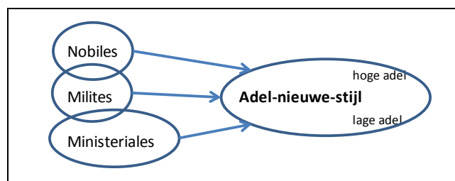
Afb. 2: Schematisch overzicht van de vervaanging van de aristocratische geledingen 1100-1300
