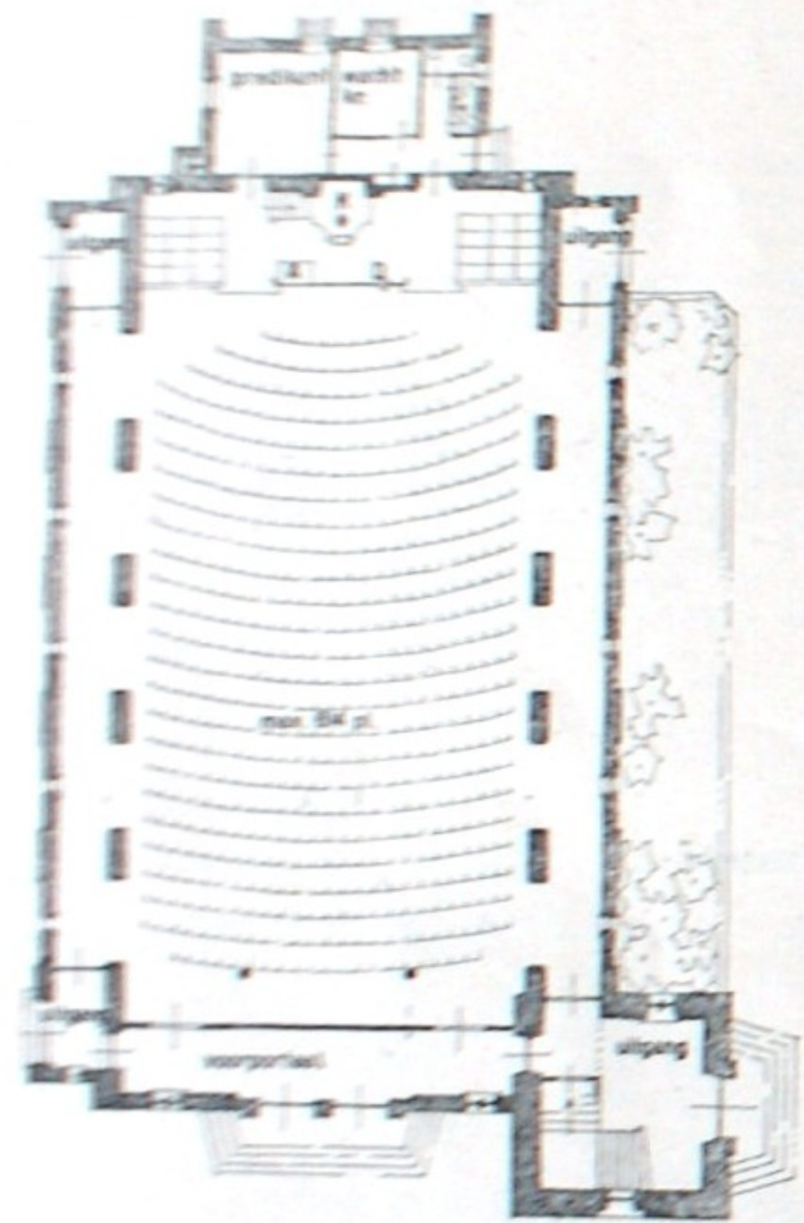
begane grond
