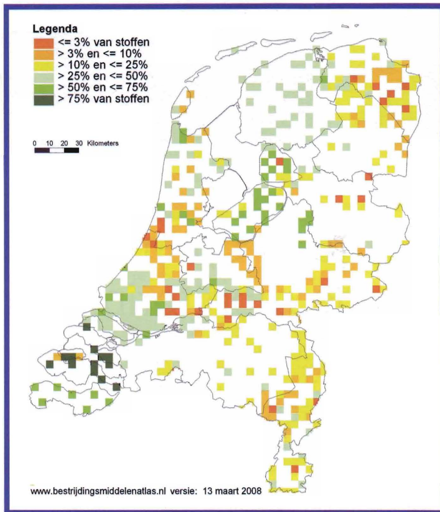
Afb. 1: Gemeten concentraties aan carbendazim getoetst aan de ecotoxicologische norm: het maximum toelaatbaar risiconiveau (MTR)
