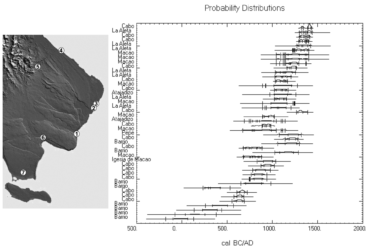
Figure 20. ^{14}\text{C} dates from: (1) El Cabo; (2) Sitio de Pepe; (3) El Barrio; (4) Punta Macao; (5) Iglesia de Macao; (6) Atajadizo; (7) La Aleta. (CALIB Radiocarbon Calibration Program, Stuiver and Reimer 1986-2005).
