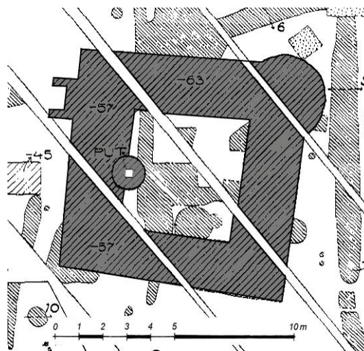
Figuur 299 Opmeting van de aangetroffen fundamenteën van Rodenburg tijdens het archeologisch onderzoek in 1939. Bron: Braat 1940, t.o. 114 Bewerking auteur.
