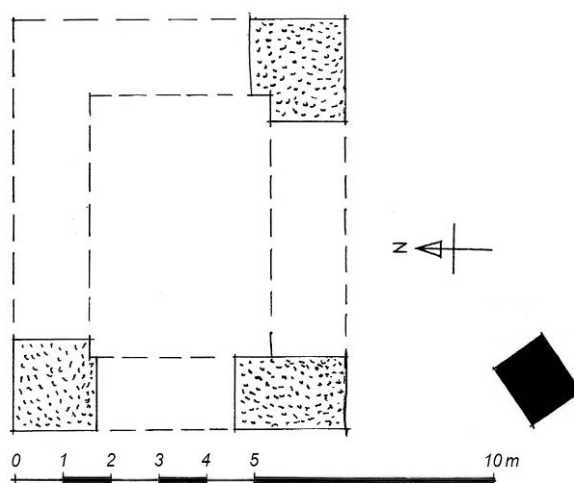
Figuur 68 Opmeting van de Joffer Achtenwoning door C. Hoek. Rechts het brok muurwerk dat tot de ringmuur zou behoren. Bron: Hoek 1965b, t.o. 5
