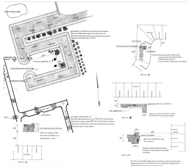
Figuur 31 Overzicht van aangetroffen funderingen van Bruëlis. Tekening B. Oele 1968. RCE, inv.nr. 1992-02449, detail
