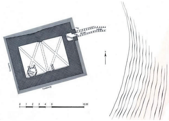
Figuur 183 Opmeting van de fundamenteën van Kathendrecht. Tekening H. van Zomeren 1963. RCE, inv.nr. 1992-07896
