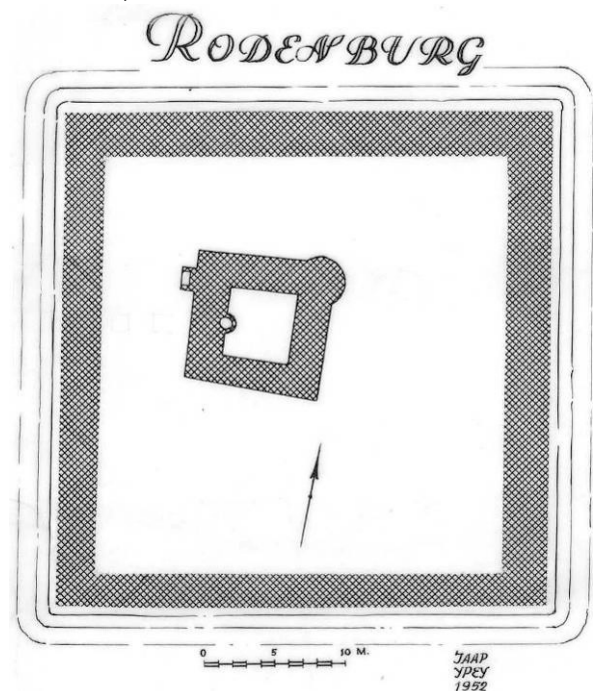
Figuur 302 Reconstructietekening van Rodenburg met ringmuur. Tekening J. Ypey 1952. RCE, inv.nr. 1991-00409
