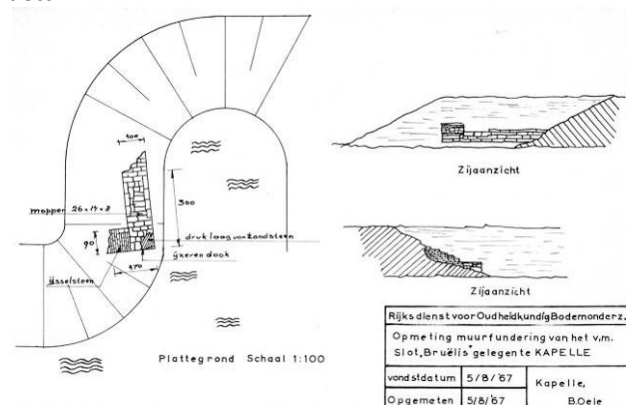
Figuur 32 Opmeting van een deel van de aangetroffen funderingen van Bruëlis. Tekening B. Oele 1967. RCE, inv.nr. 1992-02448
