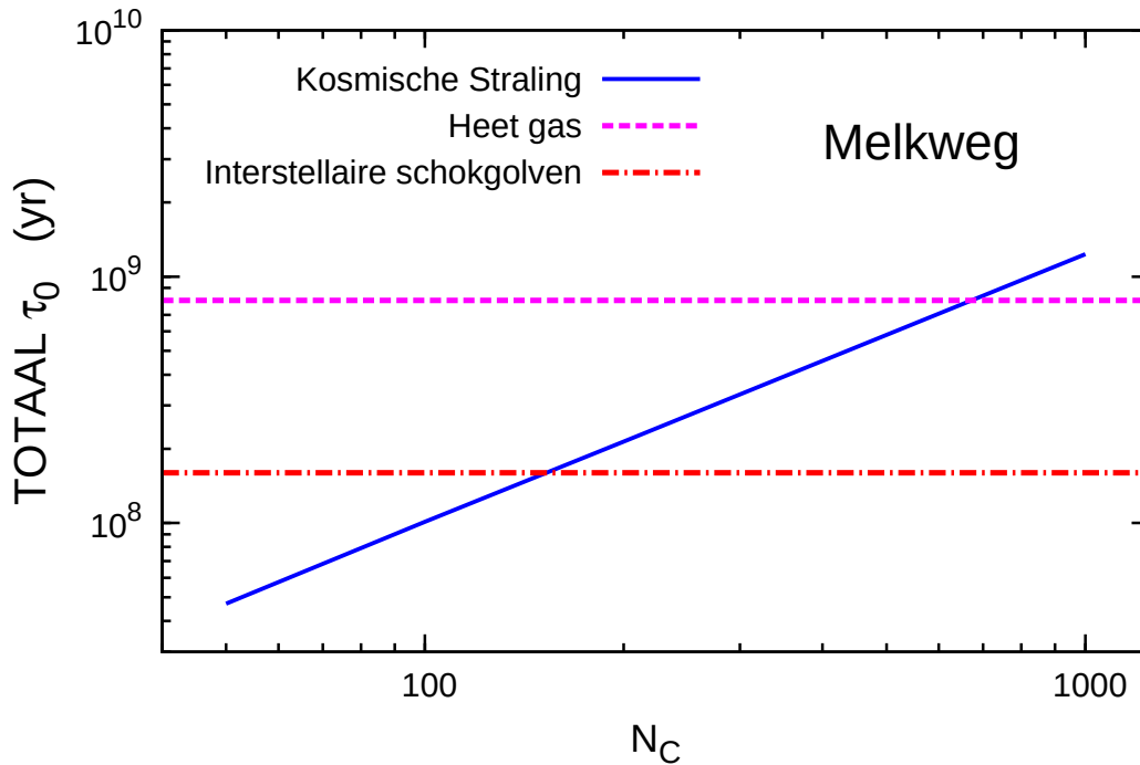
Figuur 5 — De levensverwachting van PAHs in de Melkweg ten opzichte van kosmische straling, interstellaire schokgolven ( 50 \leq v_s \leq 200 \text{ km s}^{-1} ) en heet gas dat door adiabatiscche schokgolven is verhit ( v_s > 200 \text{ km s}^{-1} ).
