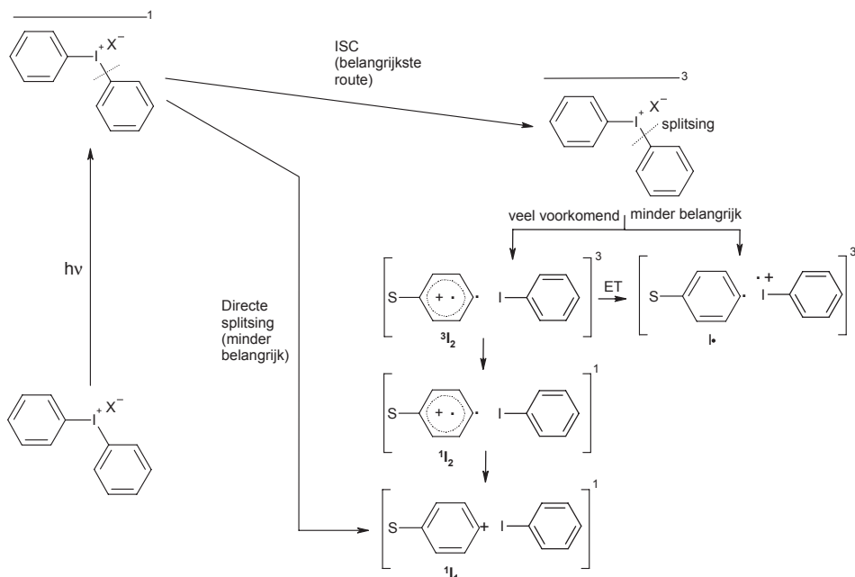
Schema 1: Het voorgestelde mechanisme van de fotolyse van difenylyjodoniumzouten.
