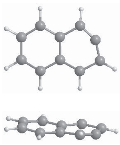
Cation ^1I_2 :
