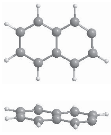
Cation ^3I_2 :
