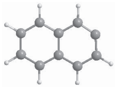
Cation ^3\text{I}_2 :
