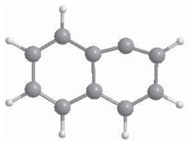
Cation ^1\text{I}_1 :
