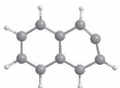
Cation ^1\text{I}_2 :
