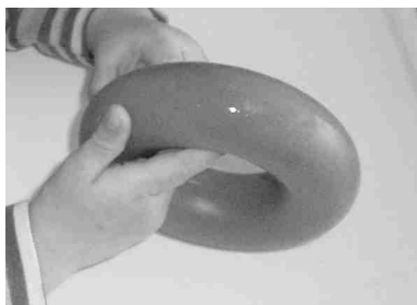
Een torus.
