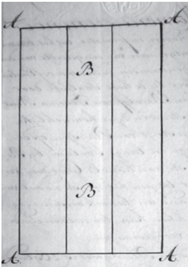
Afb. 73 Tekening van trekgraten en een legakker, door Johan Recalf van Fenema, ongedateerd. A is het te ontgronden gebied, de trekgraten, waarvan de bovenste laag aarde na de ontgroning op de middelste strook BB, de legakker, werd gedeponeerd. Na de turfwinning werd daarop hout gepoot.
