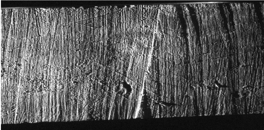
Sporen van een kraan- of raamzaag.
