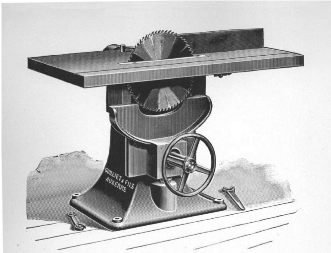
Een eenvoudige cirkelzaag. Bron: Machines à travailler le bois . Auxerre (Yonne): Guilliet & Fils, 1906, p. 135.
