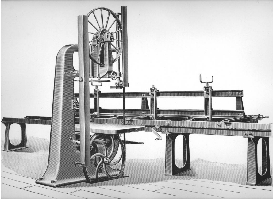
Bandzaag met slede voor het transport van een boomstam. Bron: Machines à travailler le bois . Auxerre (Yonne): Guillet & Fils, 1906, p. 60.
