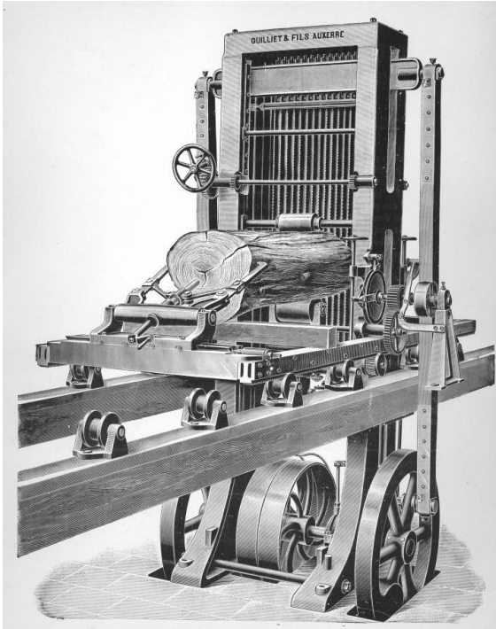
Volledig uit ijzer vervaardigde verticale raamzaagmachine. Bron: Machines à travailler le bois . Auxerre (Yonne): Guilliet & Fils, 1906, p. 28.
