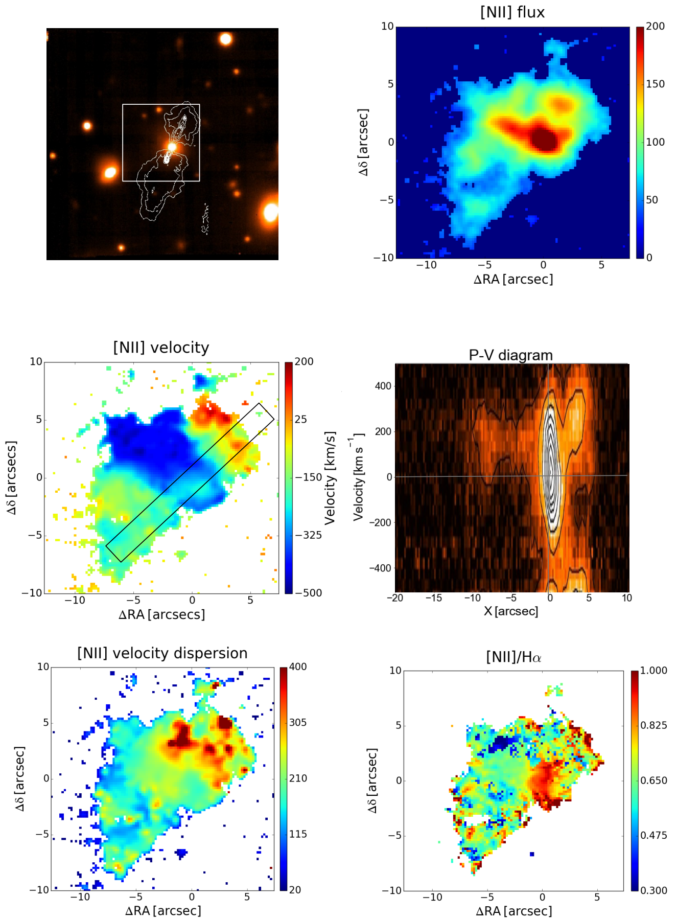
Fig. 14. 3C 424, FR II/LEG, 1'' = 2.29 kpc.
