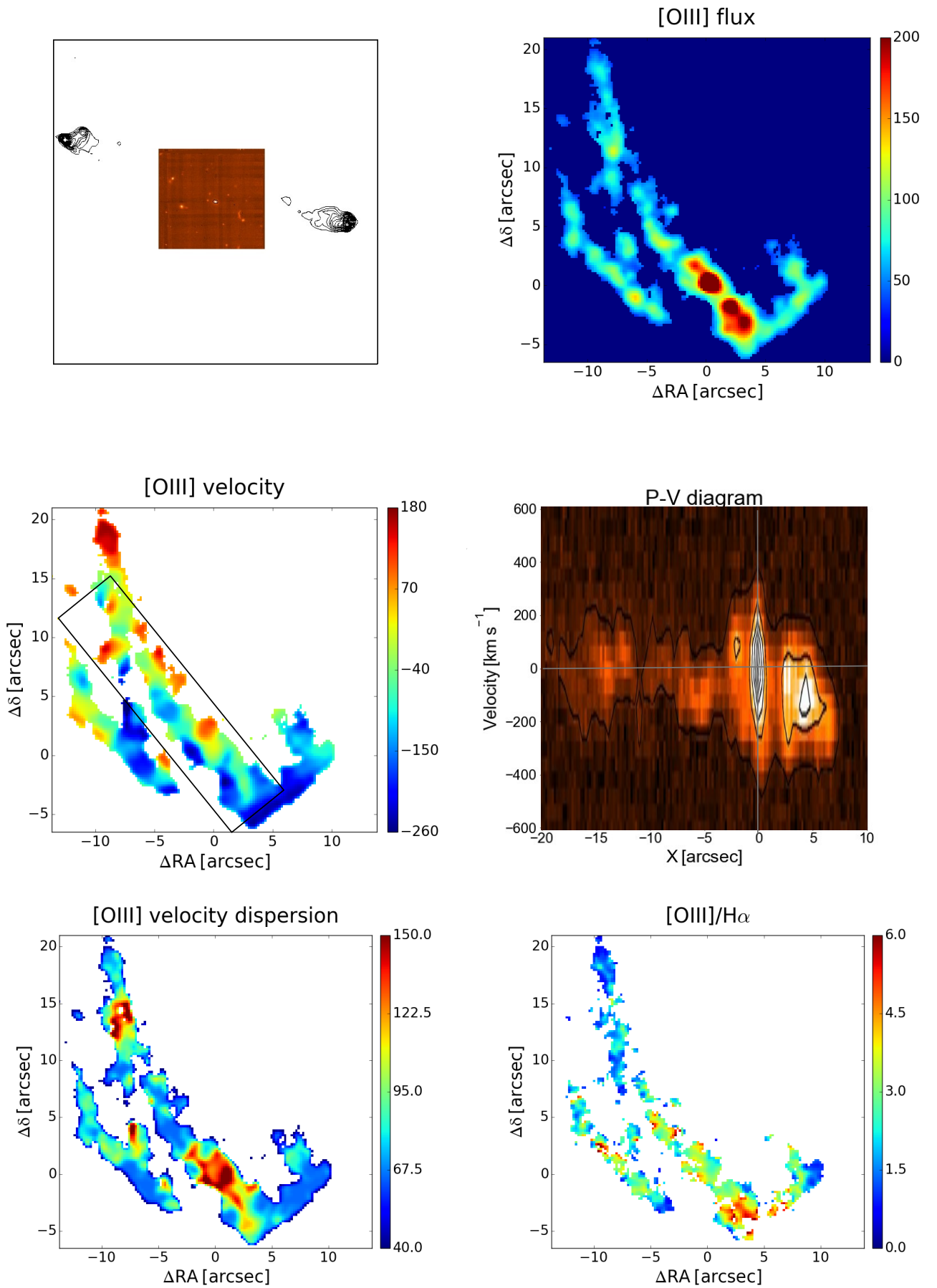
Fig. 18. 3C 458, FR II/HEG, 1'' = 4.38 kpc.
