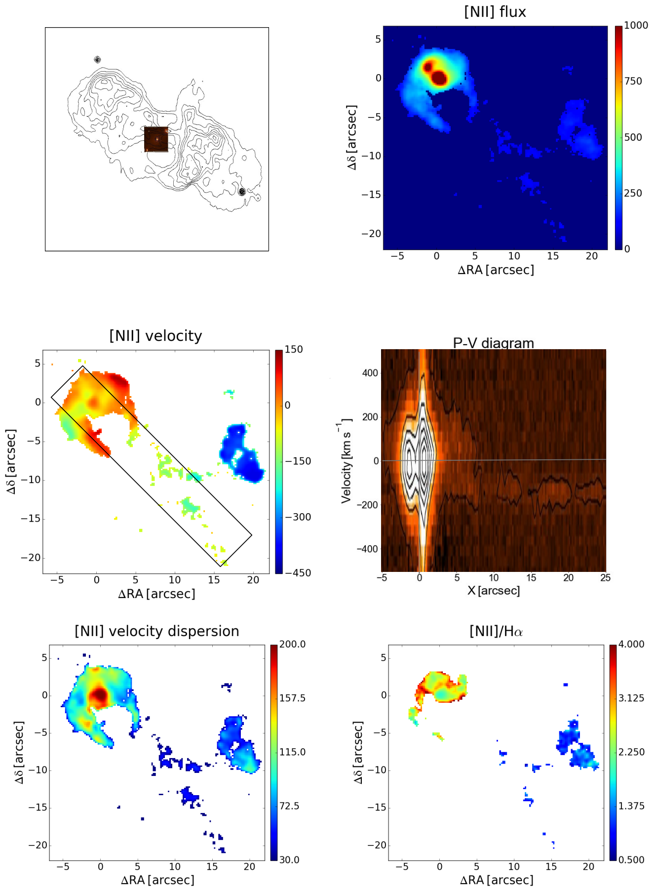
Fig. 15. 3C 442, FR II/LEG, 1'' = 0.53 kpc.
