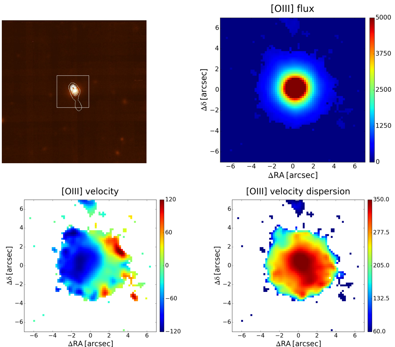
Fig. 17. 3C 456, FR II/HEG, 1'' = 3.74 kpc.
