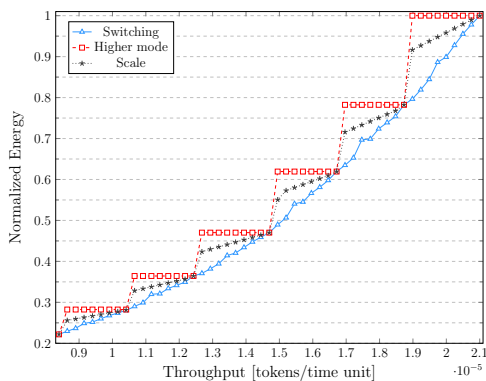
(d) DCT
