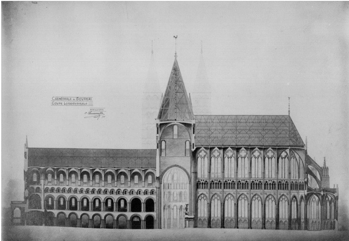
0.7A Tournai, cathédrale Notre-Dame, doorsnede in de lengterichting, Constant Sonnevillé, 1905.
