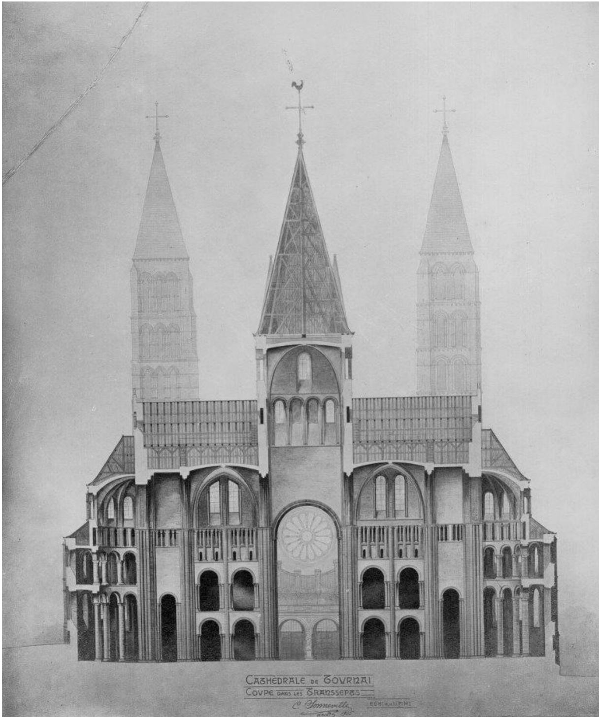
0.6A Tournai, cathédrale Notre-Dame, doorsnede over het transept richting het westen, Constant Sonnevill, 1905.
