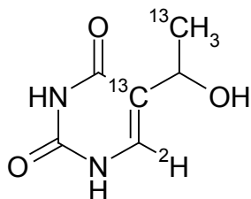
5-OH-Me-Uracil
