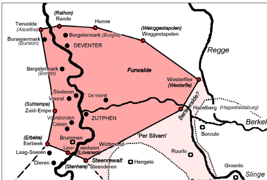
13.12: Het graafschap in Hamaland volgens de oorkonde van 1046 met de ligging van de grensplaatsen in rood. Mogelijk dat de zuidoostelijke begrenzing per silvam de dioceesgrenzen van Utrecht en Münster volgde (de lichtroze zone).
