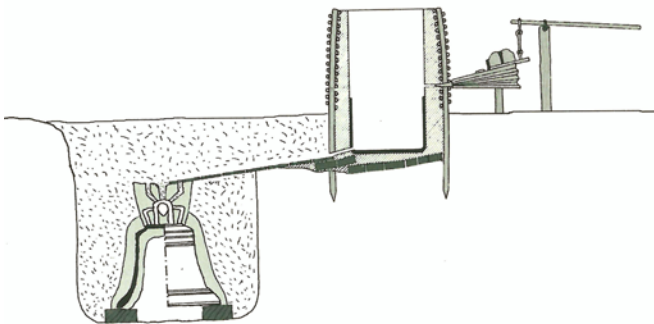
7.29: Schematische weergave van een middeleeuwse klokgietinstallatie. Rechts is de smeltoven met blaasbalg, links bevindt zich de gietkuil met de klokmal.
