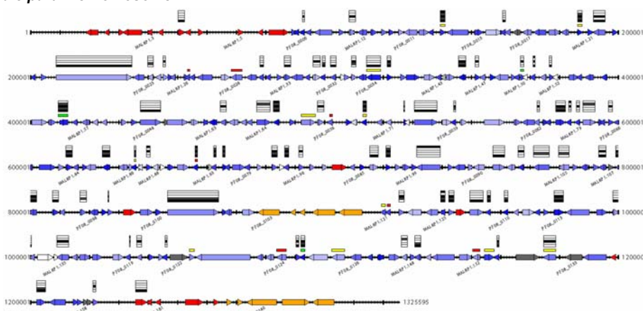
P. falciparum chromosome 8
