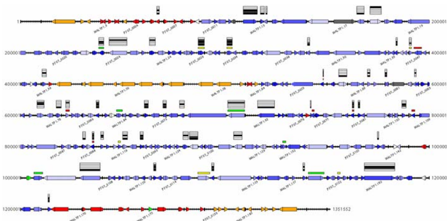
P. falciparum chromosome 7
