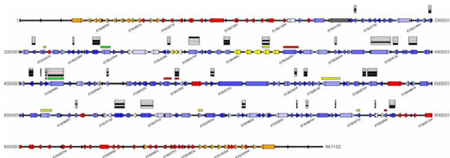
P. falciparum chromosome 2
