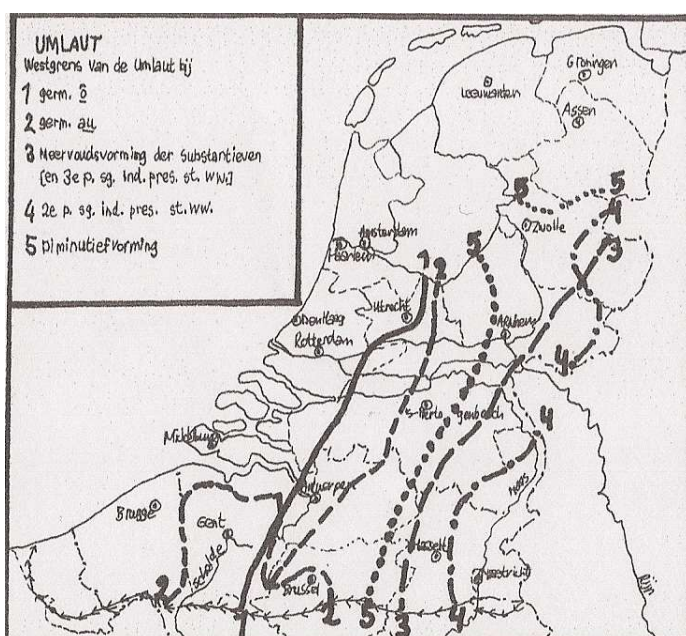
Kaart 27: Umlautsisoglossen (naar Goossens 1972)
